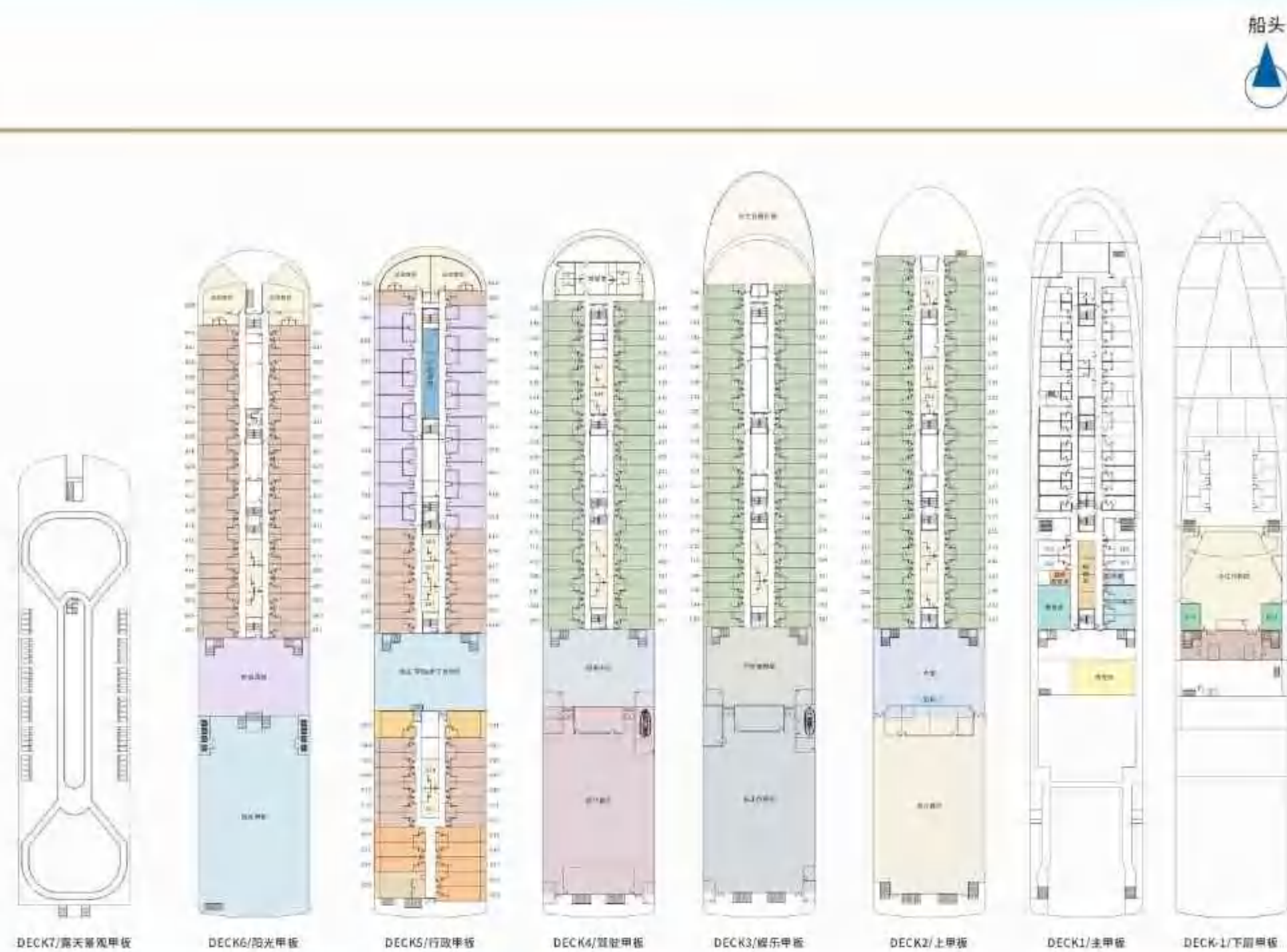
甲板平面圖
